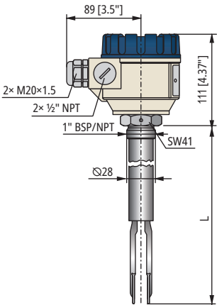
RFM / RFP-202 / 230 RFM / RFP-302 / 330
