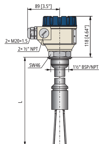
RRH / RRN-203 / 230 RRH / RRN-303 / 330
