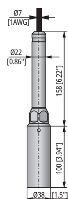
NZQ / NRQ-400 / 500 + NAZ-103
